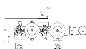
Inbyggnadsdel CO3101 (ingår ej)
