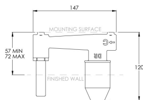
Inbyggnadsdel CO1201 (ingår ej)
