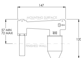
Inbyggnadsdel CO1201 (ingår ej)
