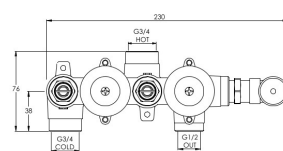
Inbyggnadsdel CO3101 (ingår ej)
