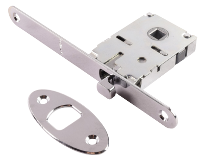
Sliding door privacy lock K1500
